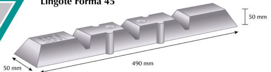
Lingote Forma 45
